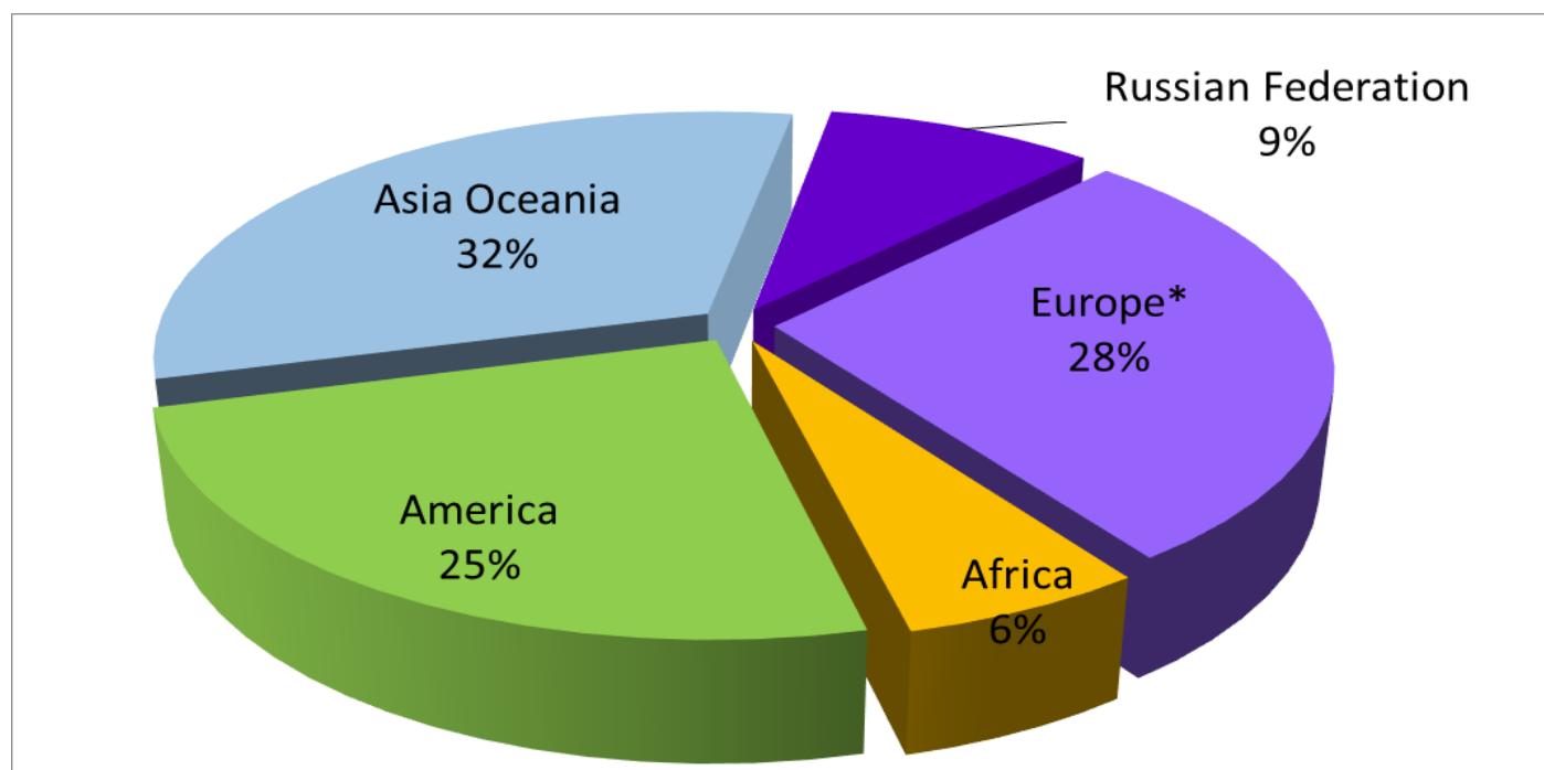
Slika 21. Dužine pruga
